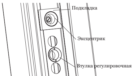
Рисунок 4 - Регулятор фалевой защелки
